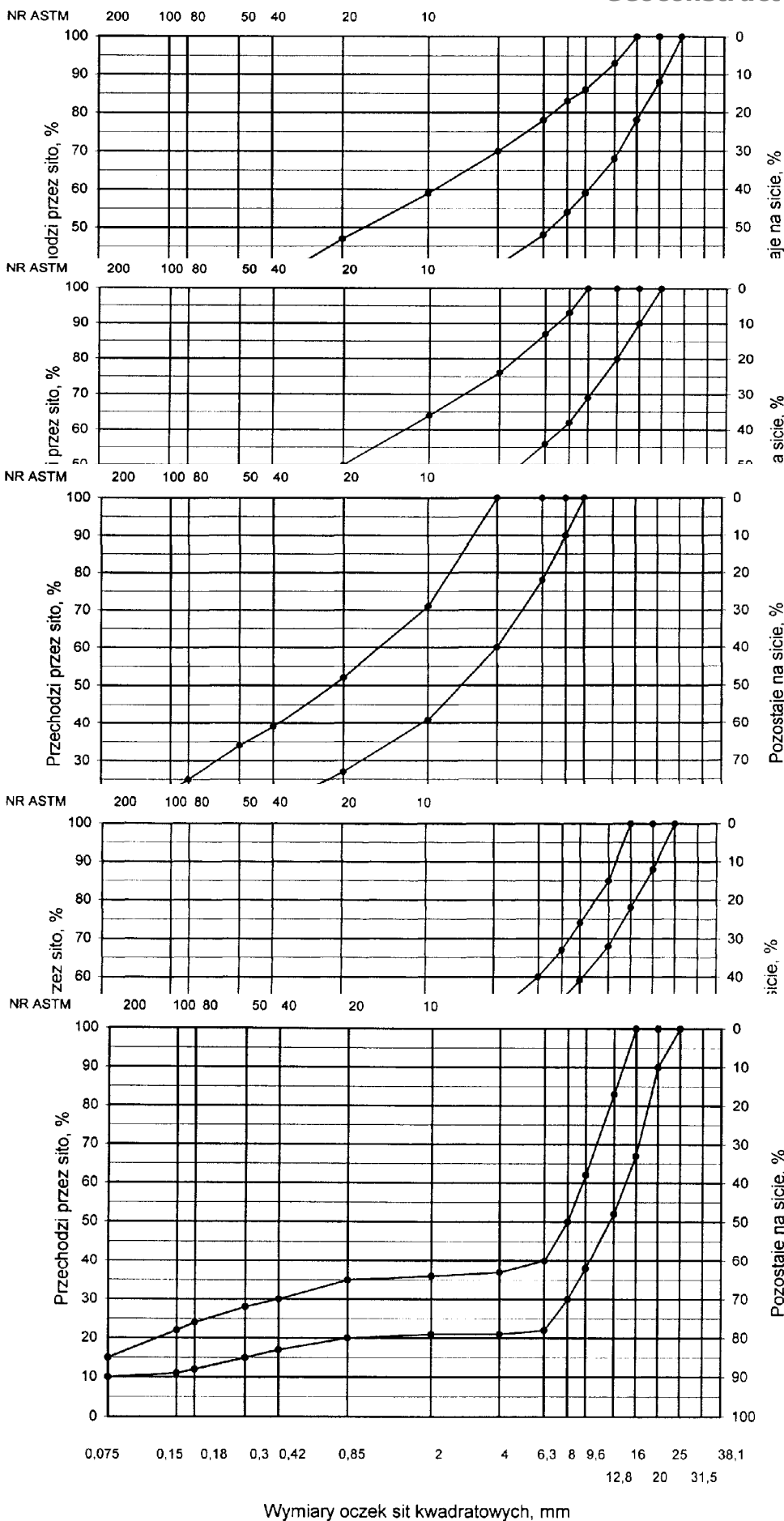
Rys. 1. Krzywe graniczne uziarnienia mieszanki mineralnej BA od 0 do 20 mm do warstwy ścieralnej nawierzchni drogi o obciążeniu ruchem dla KR1 lub KR2
