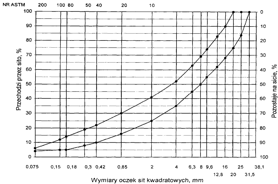
Rys. 4. Krzywe graniczne uziarnienia mieszanki mineralnej BA od 0 do 12,8 mm do warstwy wiążącej, nawierzchni drogi o obciążeniu ruchem KR1
