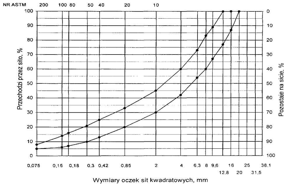
Rys. 5. Krzywe graniczne uziarnienia mieszanki mineralnej BA od 0 do 12,8 mm
