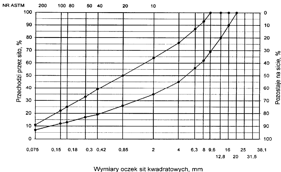
Rys. 2. Krzywe graniczne uziarnienia mieszanki mineralnej BA od 0 do 12,8 mm do warstwy ścieralnej nawierzchni drogi o obciążeniu ruchem KR1
